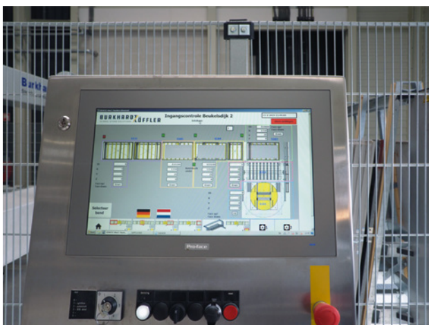
Leichte Eingangskontrolle dank Software: Auf dem Monitor sind die einzelnen (bereits von der Software eingepflegten) Platten auf einer schematischen Darstellung der Anlage identifizierbar
