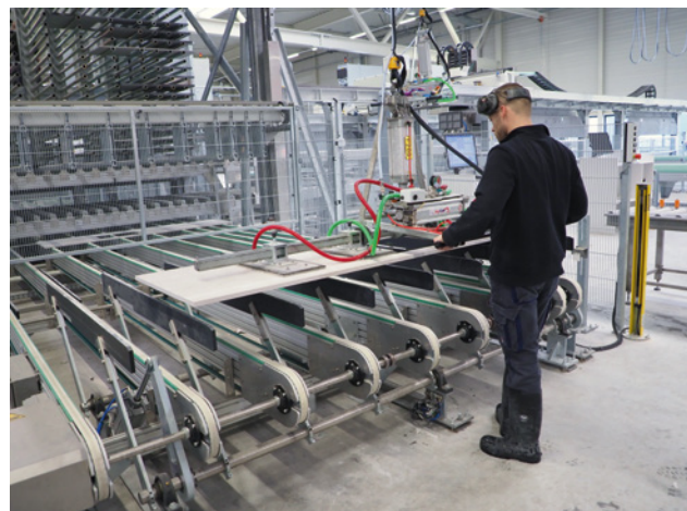
Ein Jetstone-Mitarbeiter bänkt mit dem Vakuumheber ein Werkstück von der Riemenförderstrecke ab, die ihm dieses mit ihren pneumatischen Aushüben entgegenstreckt
